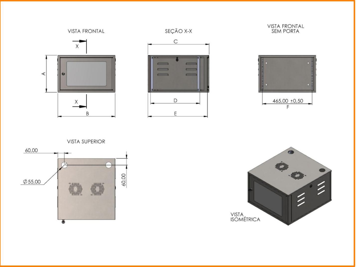
A - Altura Externa | B - Largura Externa | C - Profundidade Externa | D - Profundidade Máxima de Instalação | E - Distância entre perfis de Fixação | F - Largura de Instalação
